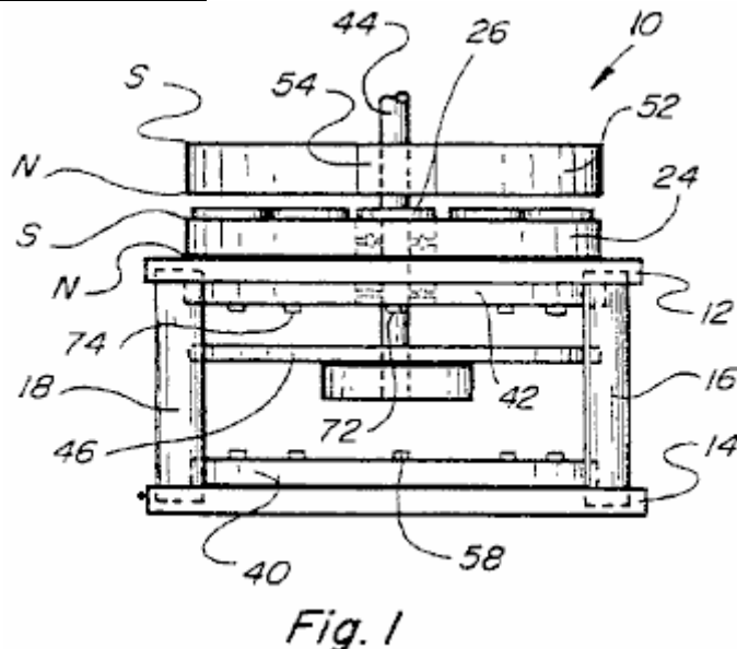
Fig.1 es una vista lateral del dispositivo impulsado de un magneticamente construido según la invención presente.
