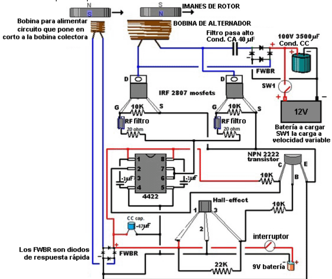
Circuito electrónico para cortocircuitar bobinas de Doug Konzen (Solo un cortocircuito por pico)
