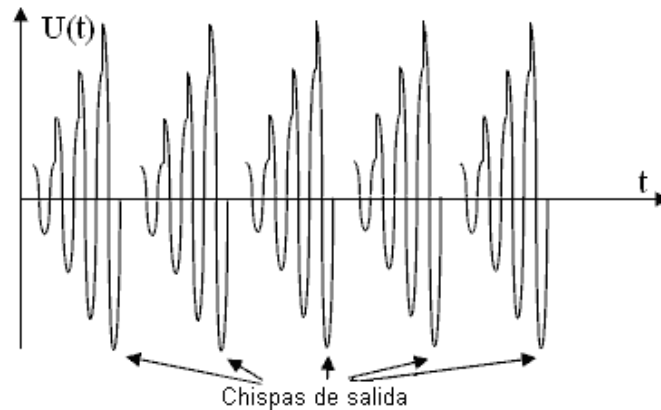
Gráfico del Generador de Excitación de Chispa
