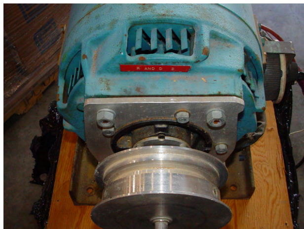
Reborde de Adaptador de Encargo Añadido a Frente de Motor
