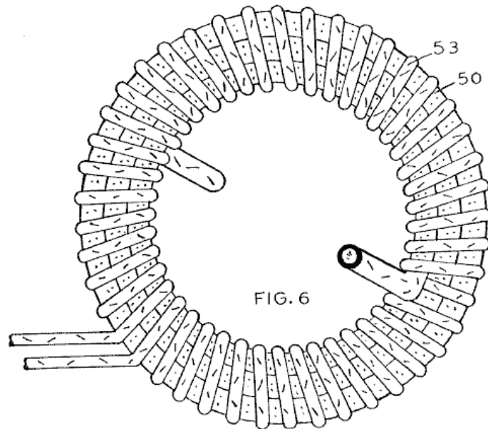
Fig.6 ilustra una configuración espiral concéntrica de la tubería 50 , con las cuerdas secundarias 53 cubierta de ello completamente.
