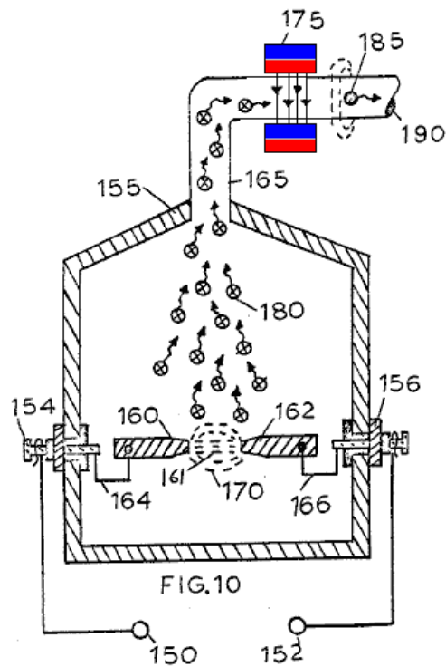
Fig.10 es una ilustración de un método alternativo de producir las partículas magnetizadas usadas en esta invención.
