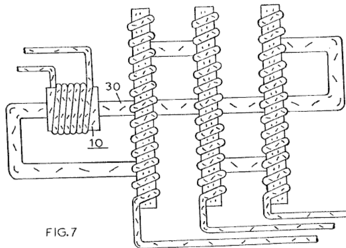
Fig.7 muestra un arreglo donde el acelerador de partículas 10 es enrollar sobre la tubería 30 del modo más o menos igual como en Fig.1 e Fig.2 . Sin embargo, en este arreglo, la tubería 30 es un lazo cerrado continuo arreglado en una configuración paralela de serie donde hay tres cuerdas secundarias que proporcionan tres salidas separadas mientras la tubería 30 carreras en serie por aquellas tres cuerdas.
