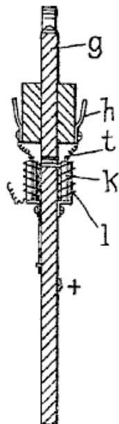
Fig. 3 es una sección a lo largo de la línea C—D de la Fig. 2.
