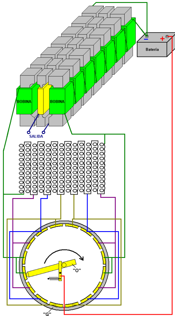
Figura 14-b. Representación esquemática completada de la Figura 14
