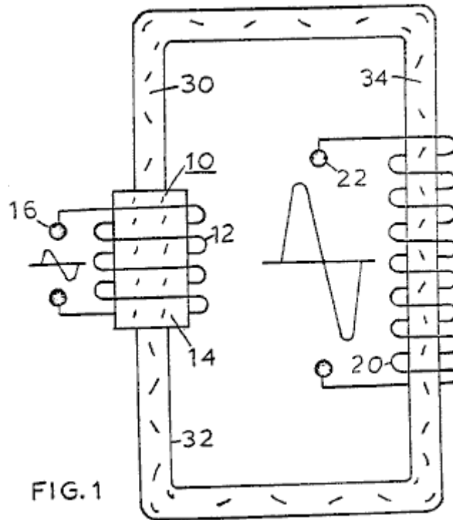
Fig.1 es una ilustración simplificada de los principios de la invención, mostrada parcialmente en el corte transversal y parcialmente ilustradamente.
