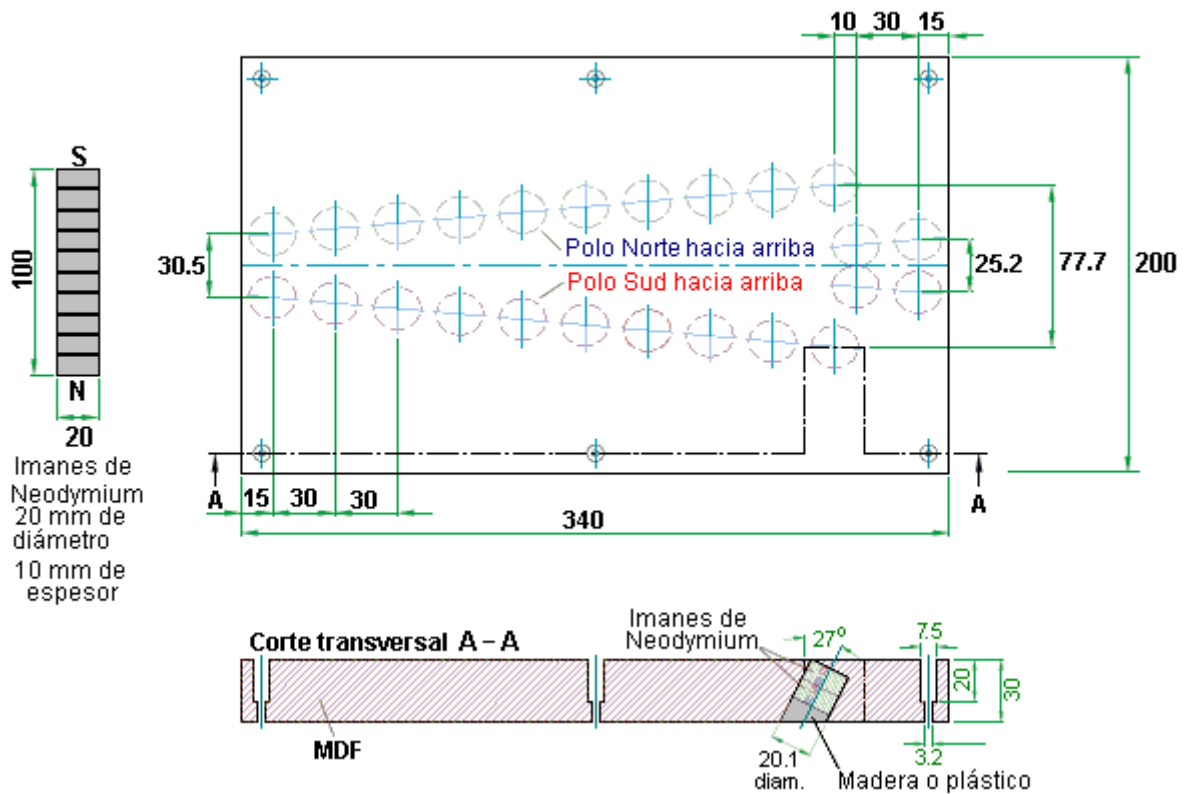
Diseño de Campo de V-acelerador de Imán Permanente por Dietmar Hohl, 6 de abril 2007
