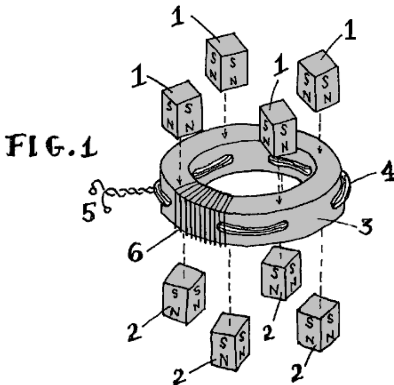
Fig.1 vista explotada del generador de esta invención.
