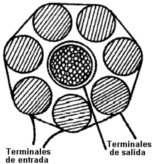
Fig. 28 Vista superior de generador Hubbard
