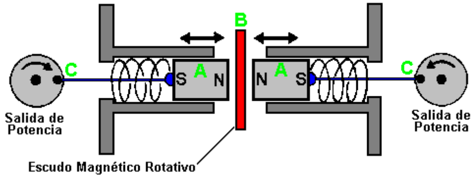
Diagrama del 2do estilo de operación del motor de John W. Ecklin
