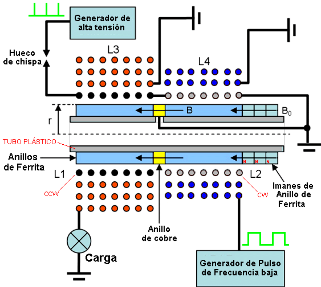
Fig.1 Corte transversal del bobina de ejemplo. Algunos detalles de realización actuales pueden diferenciarse del arreglo mostrado encima, pero esto no cambiará la operación de dispositivo. Este diagrama no debe escalar.
