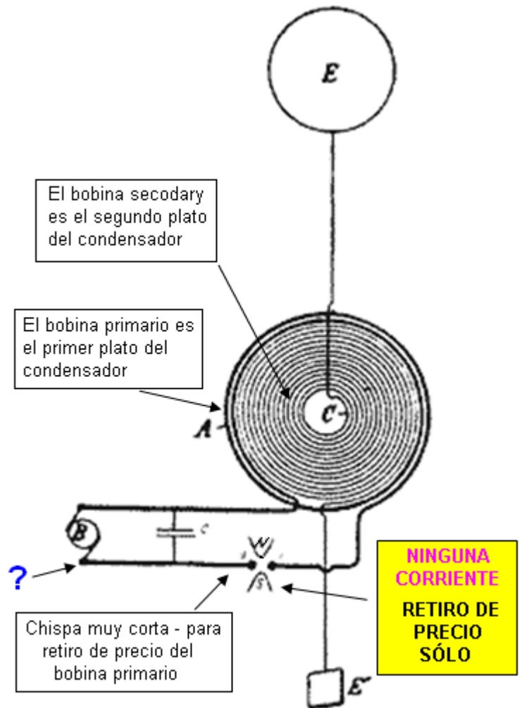
El Transmisor de Ampliación de Tesla
