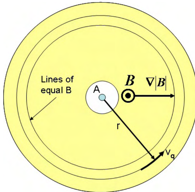
Fig.2. Giro de la partícula cargada emitida en el declive del campo magnético en un disco (p.ej latón) en la condición de resonancia de ciclotrón. El disco gira en dirección contraria a las partículas.
