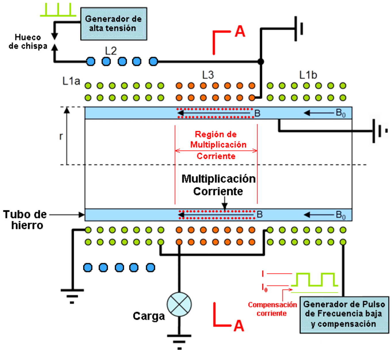
Fig.2 Este es un tubo de Hierro bobina de ejemplo basado. El arreglo de los bobinas en el tubo es diferente en varias realizaciones del dispositivo. Este dibujo no debe escalar y el grosor de la pared de tubo es exagerado.
