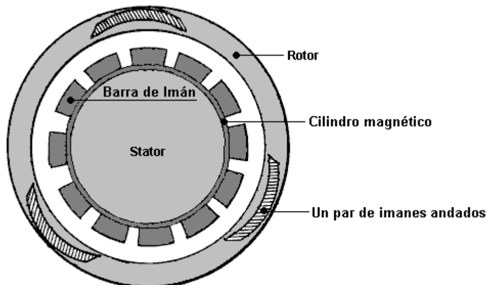
Note que los huecos entre los imanes de pista no son una anchura constante
