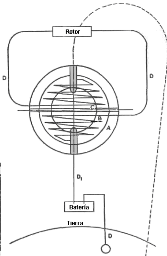
Salido: Inventor Karl Schappeller el Derecho: el el del el Dispositivo de Karl Schappeller. A. Acero la cubierta exterior. B. Forro cerámico especial en que los tubos son inc luido. C. El centro sin substancia, llenó por el magnetismo brillando cuando en el funcionamiento. D. Los tubos, circuito y terrícola.
