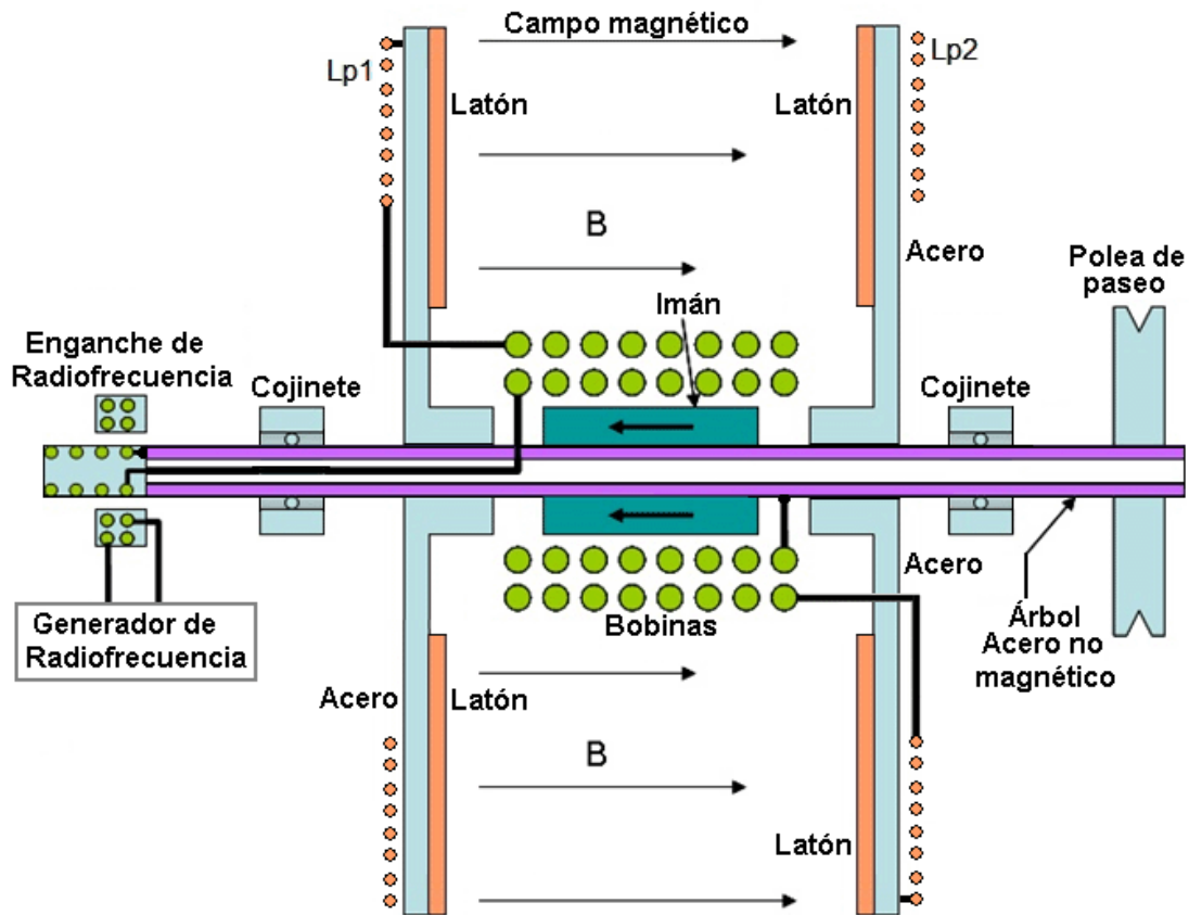
Fig.1 El corte transversal del dispositivo parecido a un ciclotrón dual
