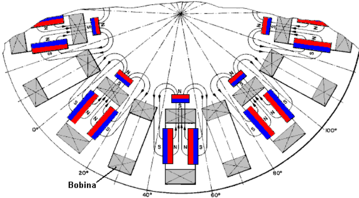
Diagrama del "Carousel" Moto-Generador de Imán Permanente
