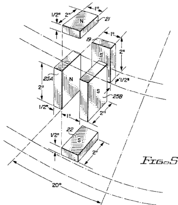
Detalle del Montaje de Imanes del Moto Generador Carousel
